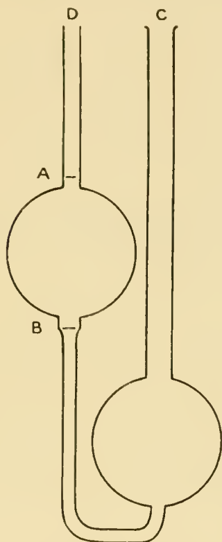
FIG. 97. GLASS VISCOSIMETER
