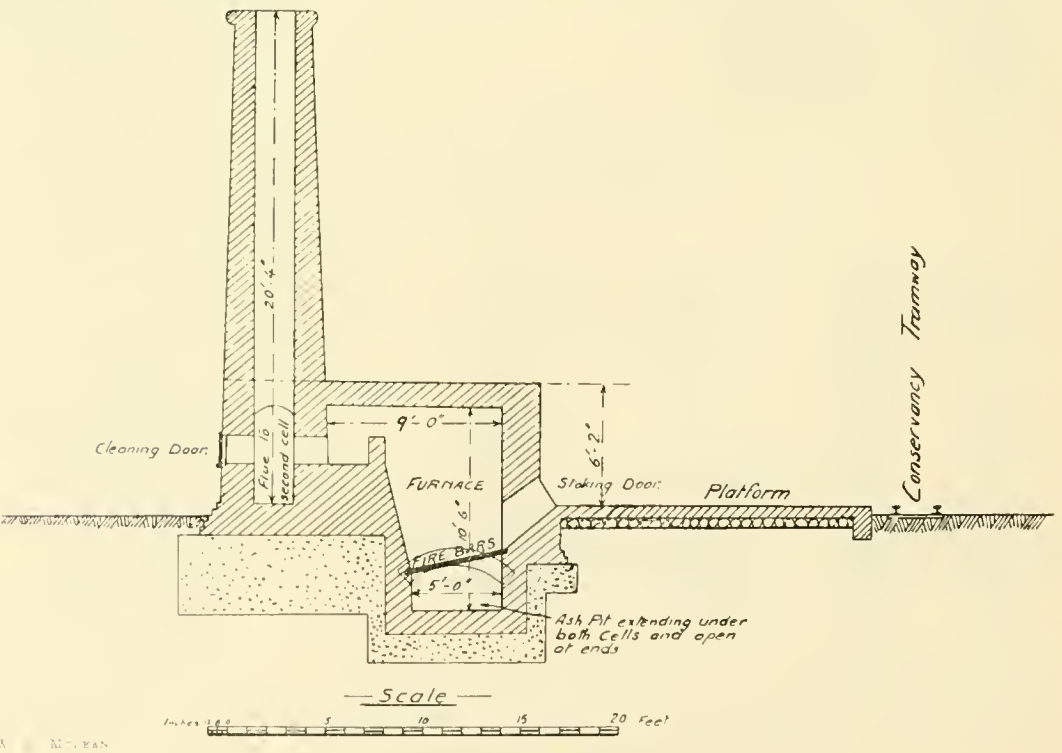
FIG. 97.—Refuse destructor
