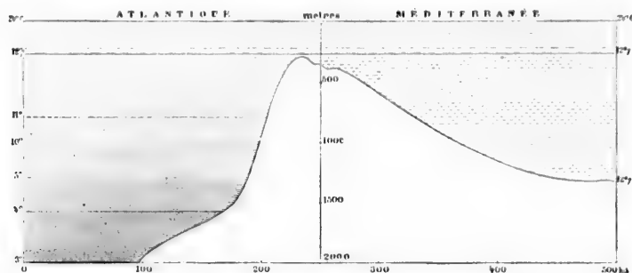
N° 3. — TEMPÉRATURE DES EAUX PROFONDES DES DEUX CÔTÉS DU DÉTIL DE GIBRALTAR.
