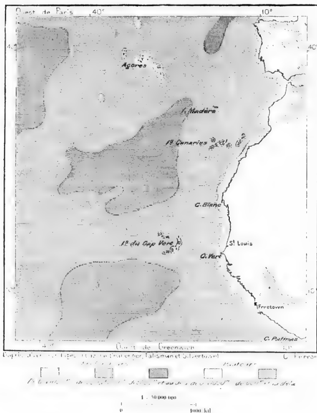
5° 1. — PROFONDEURS DE L'ATLANTIQUE AFRICAINE.
