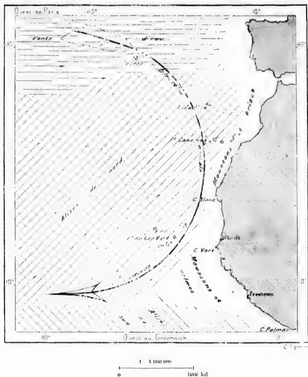
N° 3. — VENTS ET COURANTS DE L'ATLANTIQUE.
