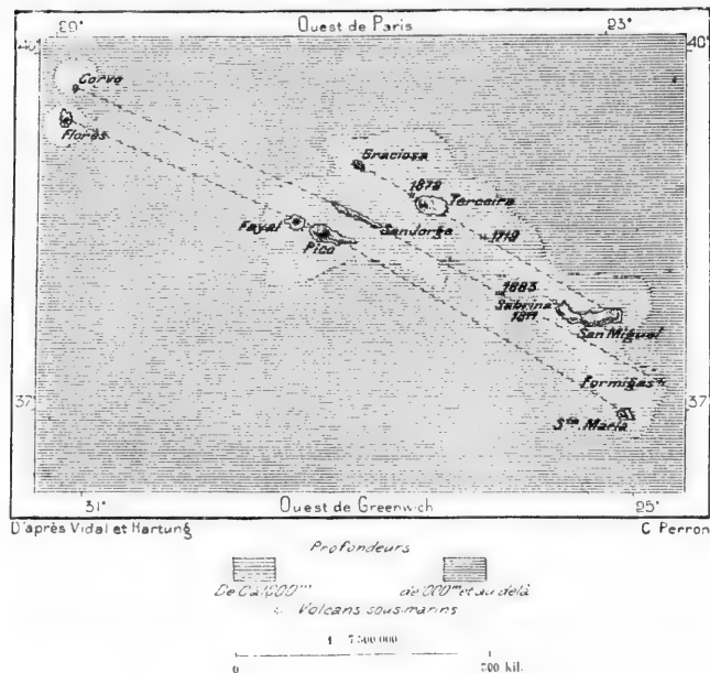
N° 5. — ALIGNEMENTS VOLCANIQUES DES AÇORES.
