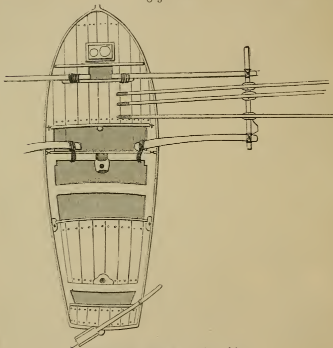
Dongolanische Nilbarte von oben gesehen.
